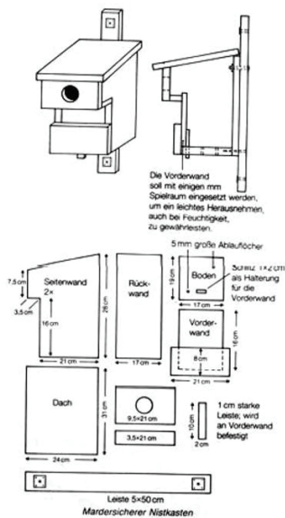
Bild: Der Nistkasten als Explosionszeichnung.
